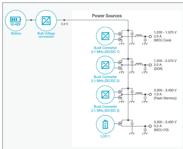
图 8. 汽车信息娱乐供电系统示意图。
