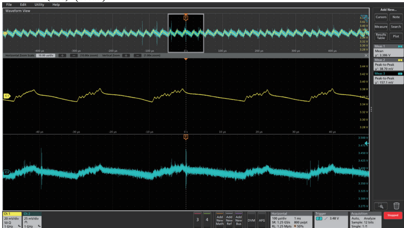
图 6. 通道 2 (蓝色迹) 显示了传统 10x 无源探头的峰峰值噪声为 157.1 mV, 在通道 1 上使用泰克 TPR1000 低噪声纹波探头时的峰峰值噪声则为 38.7 mV (黄色迹)。
