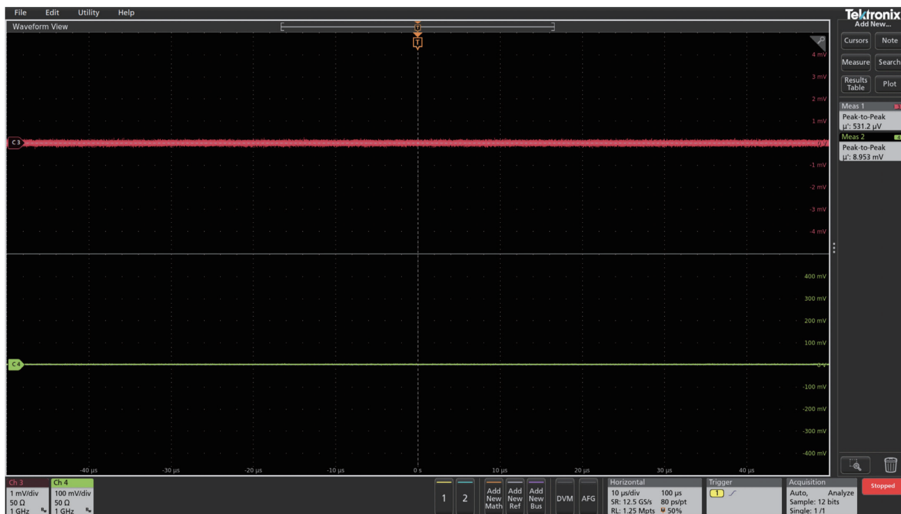
图 7. 垂直标度对测得随机噪声的影响。这两条通道都没有连接输入。通道 3 在 1 mV/div 时的峰峰值噪声为 521.2 μV，通道 4 在 100 mV/div 时的峰峰值噪声为 8.953 mV。这比通道 4 上报告的噪声多出来大约 17 倍。注意，对通道 4，8.953 mV 不到满刻度电压的 1%。
