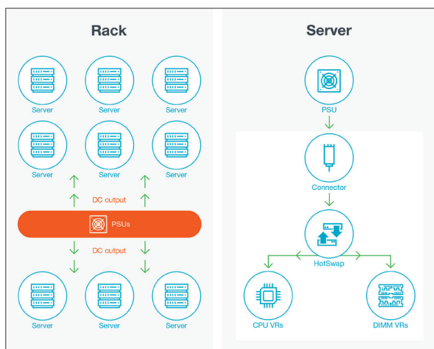
图 9. 服务器供电系统示意图。
