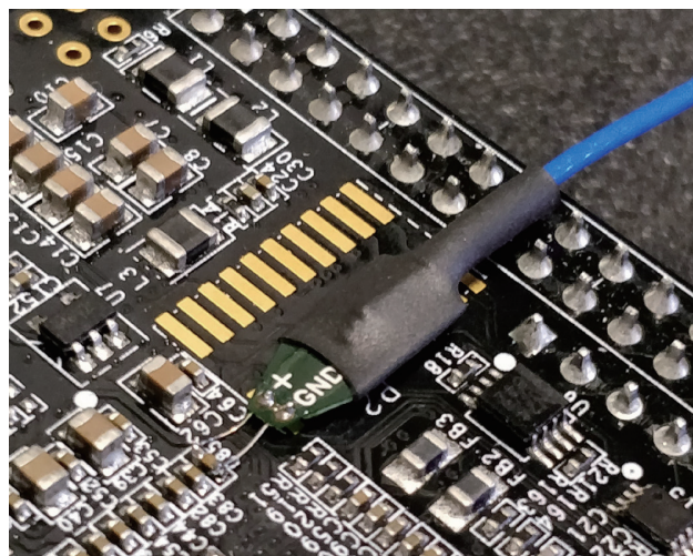
图 4. 透过 0402 解耦电容器连接的 TPR4SIAFLEX 焊接转接头。
