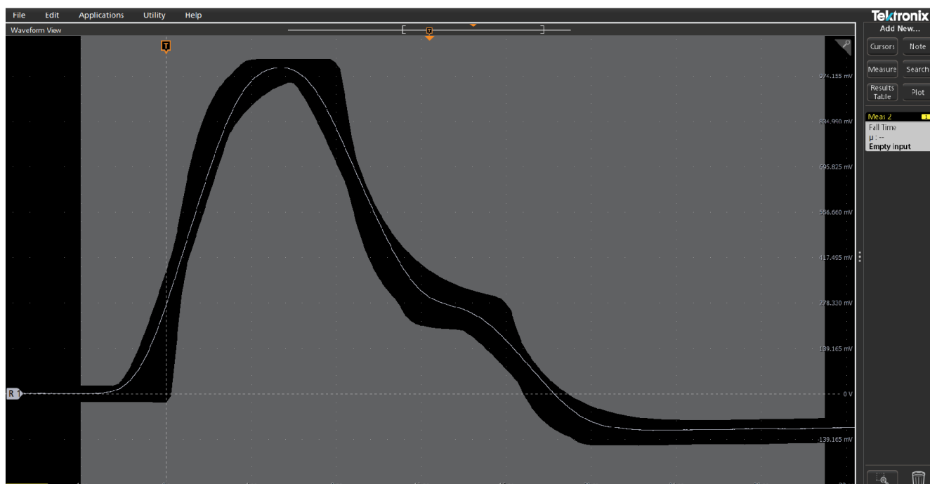
TekExpress 以太网，运行 1000BASE-T 模板测量
