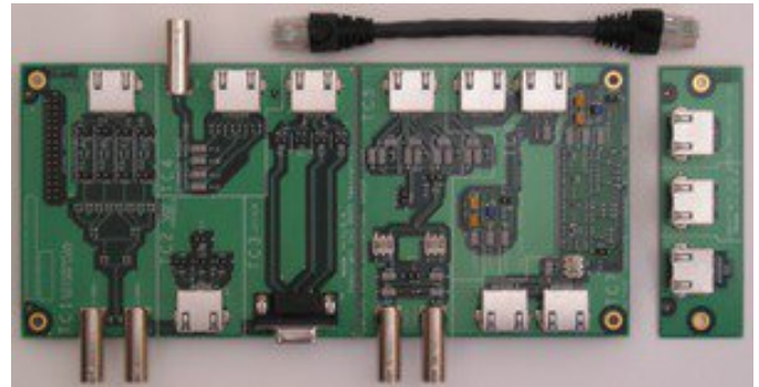
TF-GBE-BTP 基本以太网测试夹具。
