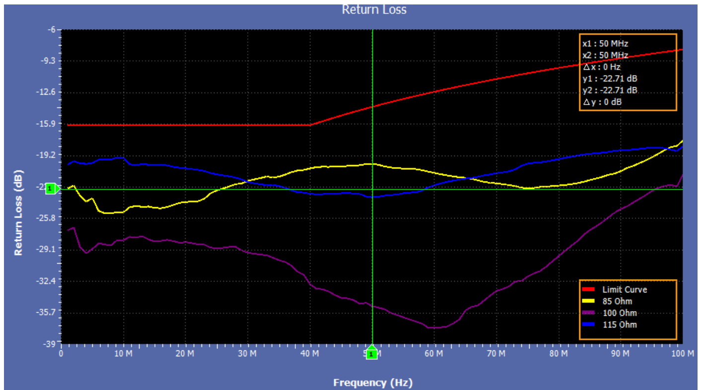
1000BASE-T 回波损耗绘图
