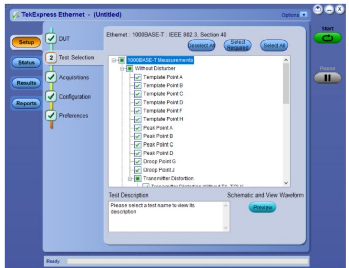
TekExpress 以太网测试选择面板
